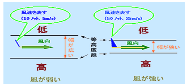
(図2) 等高度線間隔と風速
