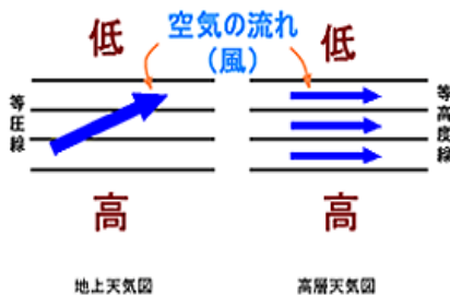
(図1) 等圧線、等高度線と空気の流れ(風の吹き方)
